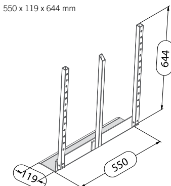
Standard 12 cm - Montants rallongés 550 x 119 x 644 mm
