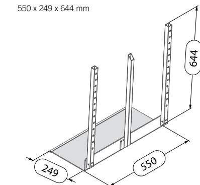
25 cm - Montants normaux 550 x 249 x 644 mm
